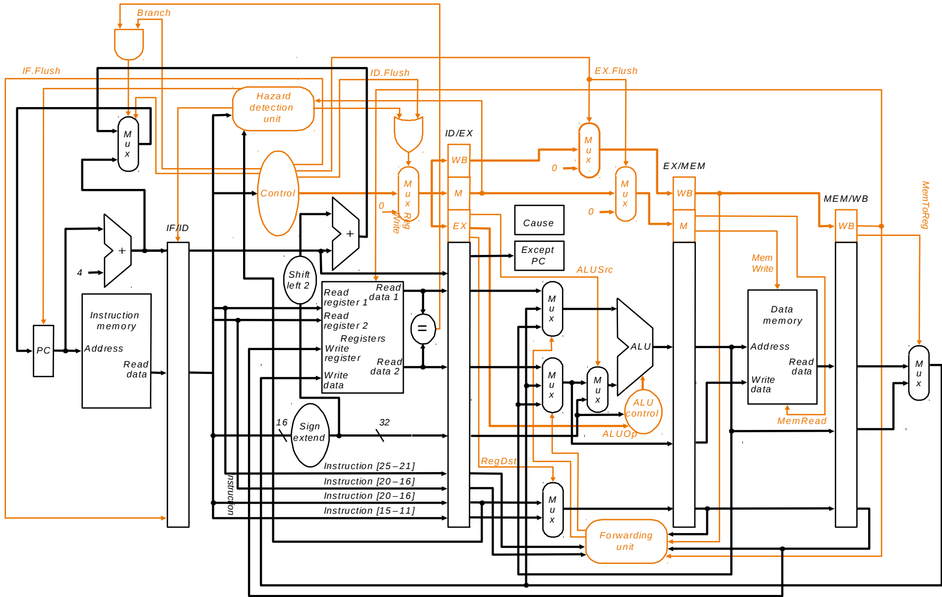
Datapath MIPS con Soporte para Pipeline.
